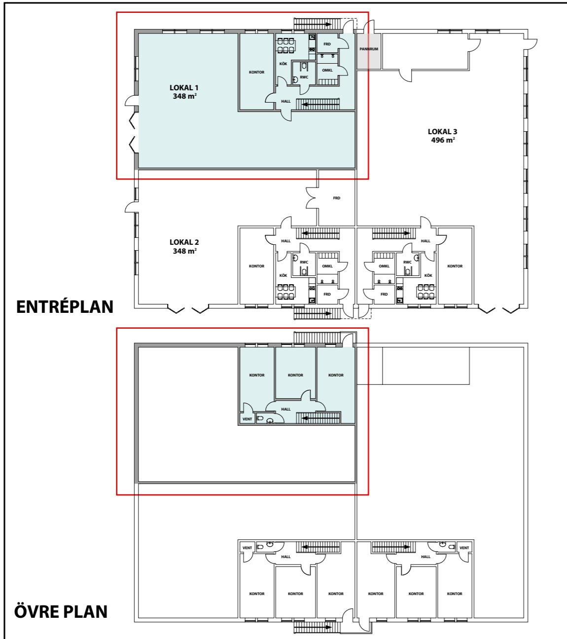
ENTRÉPLAN
