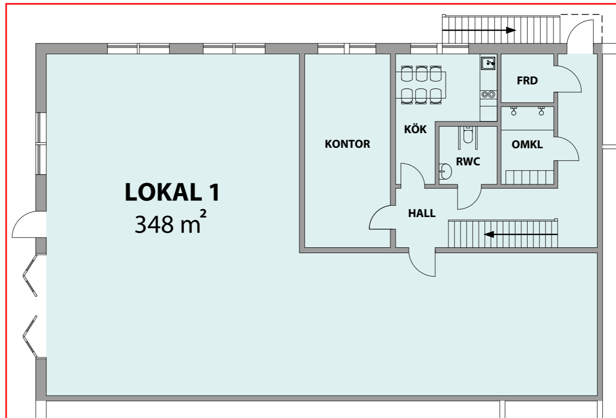
ENTRÉPLAN
