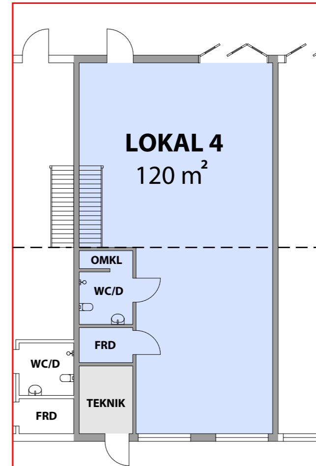
ENTRÉPLAN
