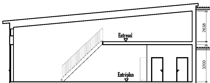
SEKTION
